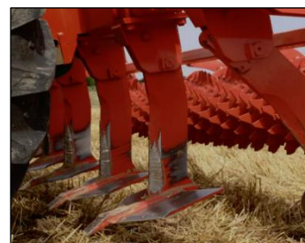
Abb. 2: Untergrundhaken
